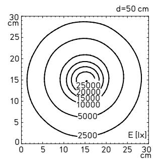
Beleuchtungsstärke mit 10°-Optik
