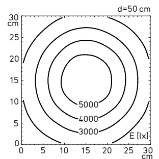
Beleuchtungsstärke mit 40°-Optik
